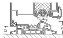
Bezbariérový práh s přerušným tepelným mostem do výšky 20 mm
