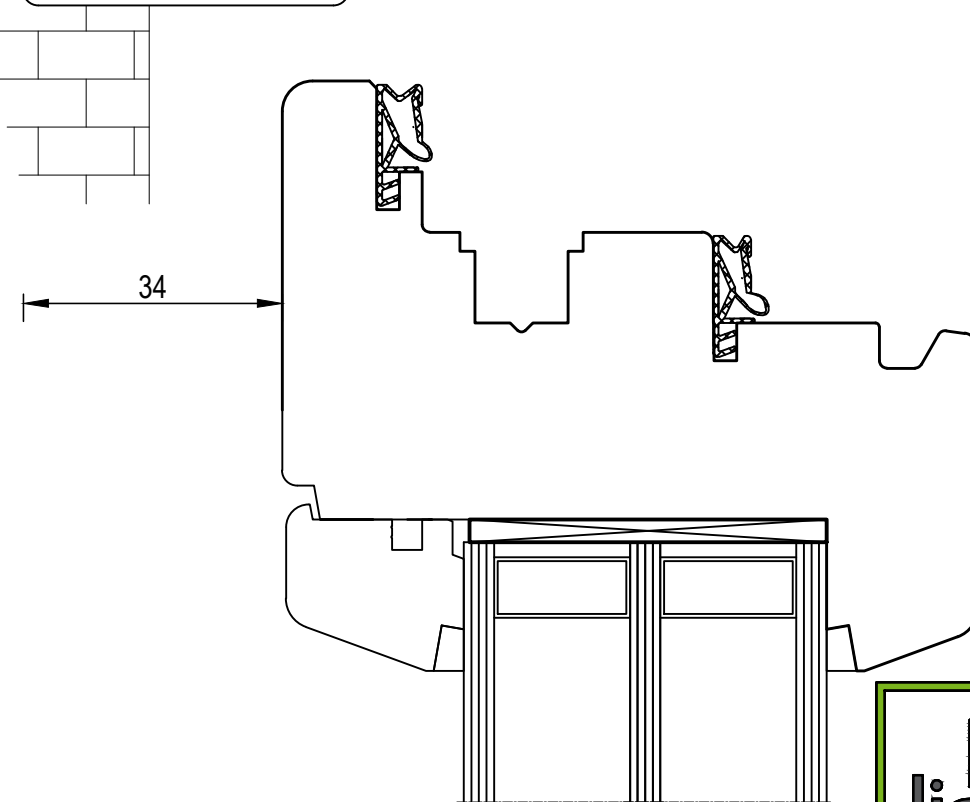
Geometrie otevření se skrytým kováním MACO Multi Pover
