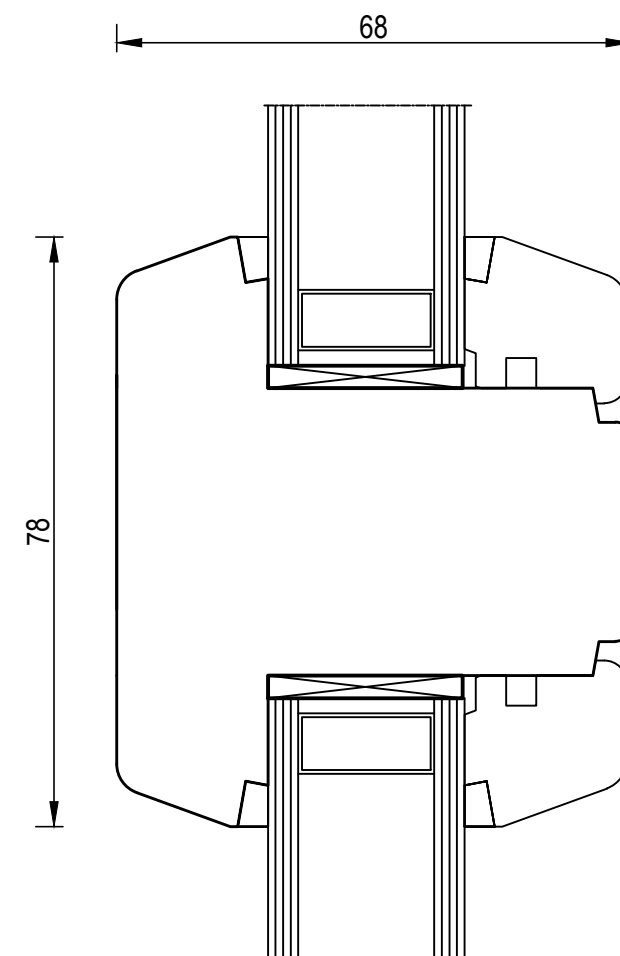
Sklodělicí příčka vodorovná 78mm
