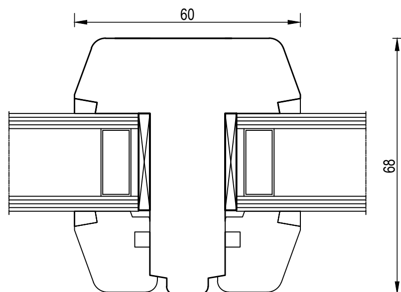
Sklodělicí příčka svislá 60mm
