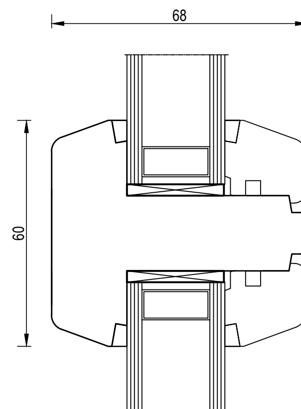
Sklodělicí příčka vodorovná 60mm
