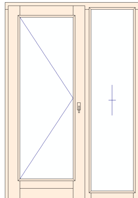
Jednokřídlé fix vpravo
